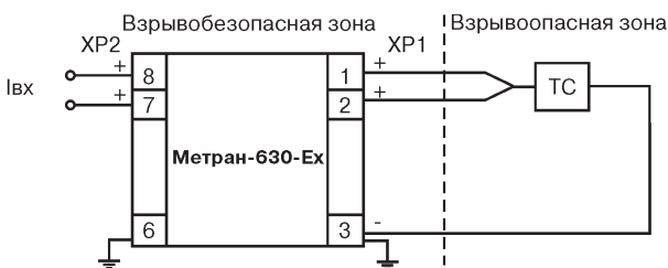
Метран-630-105-Ех
