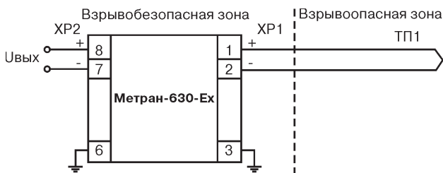
Метран-630-101-Ех, Метран-630-102-Ех
